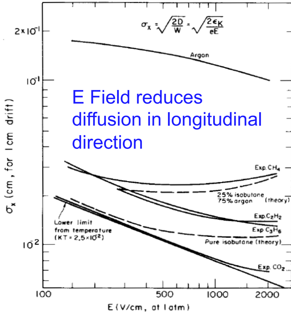
Difusión longitudinal en función del campo E
