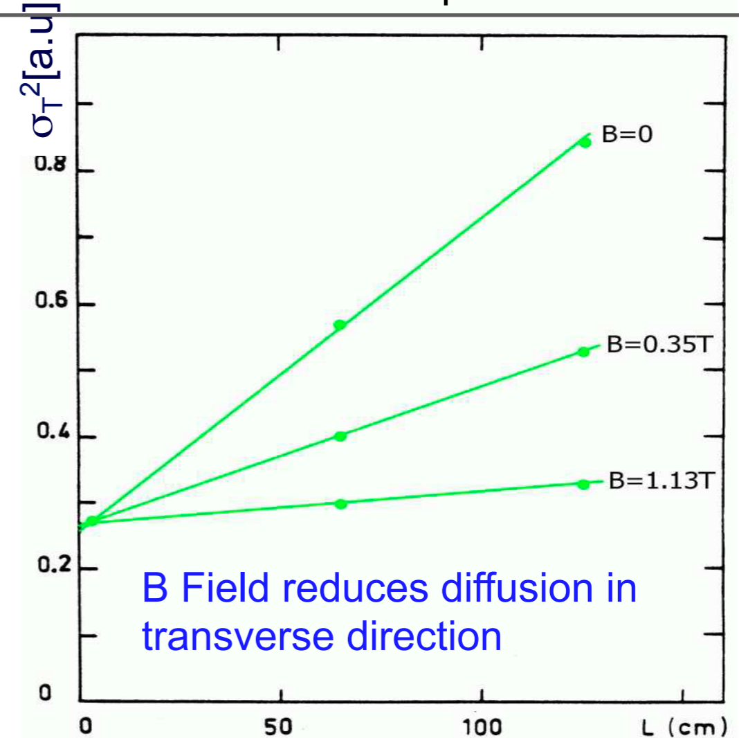
Difusión transversal vs longitud de deriva para diferentes campos B
